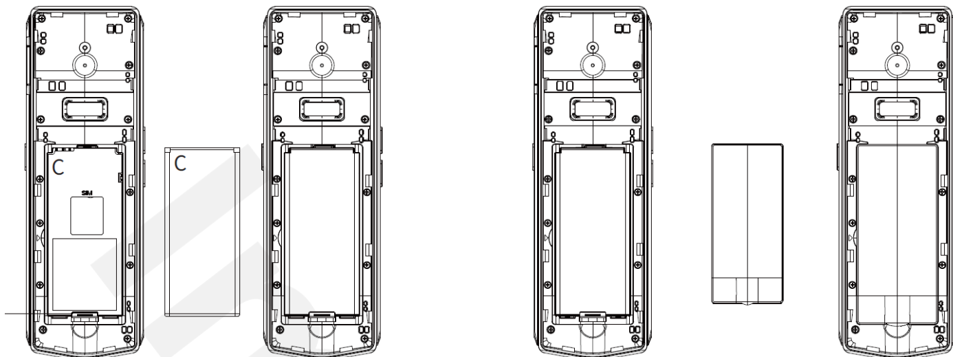
Instalacija baterije
